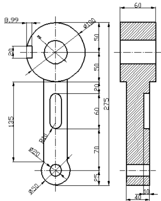
2D výkres
