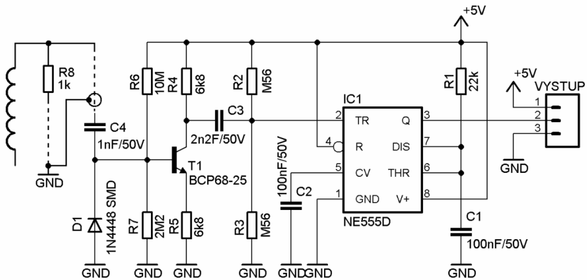
Obr. 4.6 Schéma zapojení otáčkoměru
